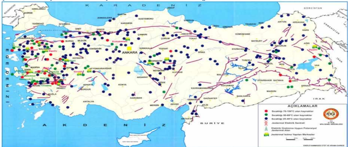
Şekil 11: Türkiye Jeotermal Kaynak Alanları ve Sıcaklık Dağılımı Haritası
