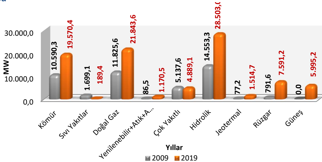
Şekil 3: 2009 ve 2019 Yılları İçin Birincil Enerji Kaynaklarına Göre Türkiye Kurulu Gücü
