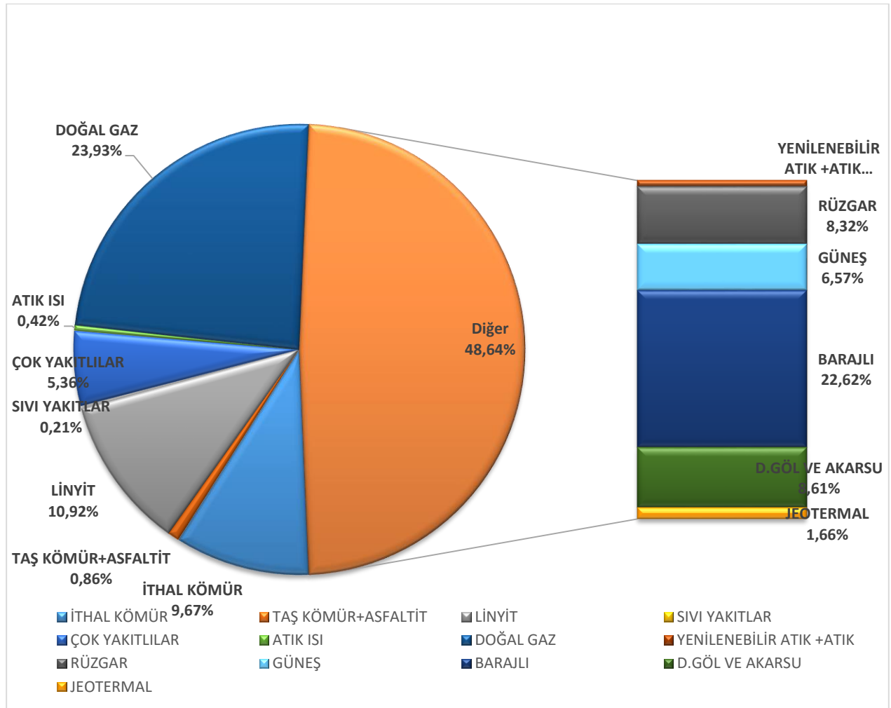
Şekil 1: 2019 Yılı Kurulu Gücünün Birincil Enerji Kaynaklarına Göre Dağılımı (MW)
